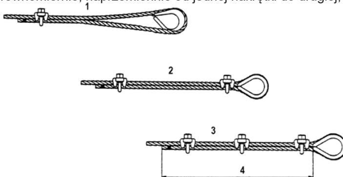
Rysunek 1 - Kolejność montażu zacisków
